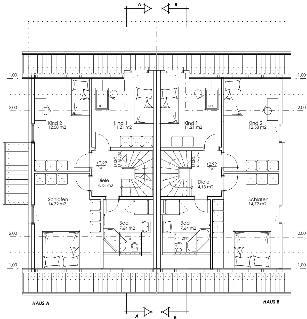
DACHGESCHOSS
